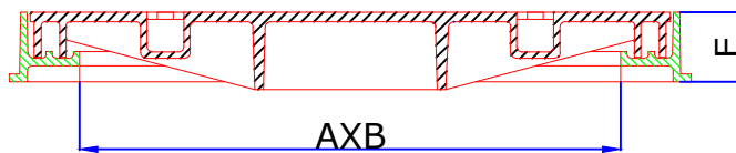
SECTION - A-A'
